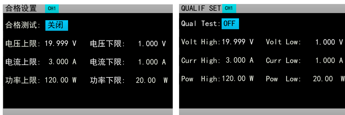
图 2.14.1 合格测试设置界面
