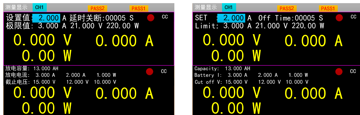
图 2.14.2 开启合格测试后的界面
